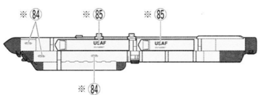
《AN/ALQ-184 ECM ボッド (レーダー波ジャミング装置)》 AN/ALQ-184 ECM Pod
